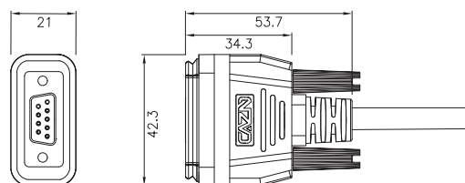
尺寸图 DIMENSIONS
